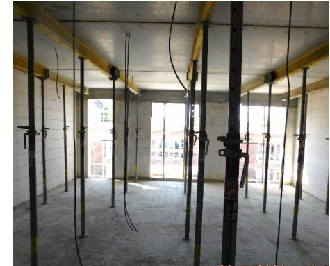
Wohnung im ersten Obergeschoss
